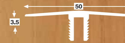
LLT22 TWIN
