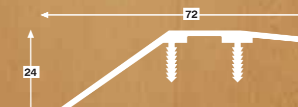
FR3 22 RAMP
