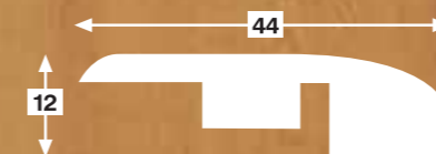
HR RAMP
