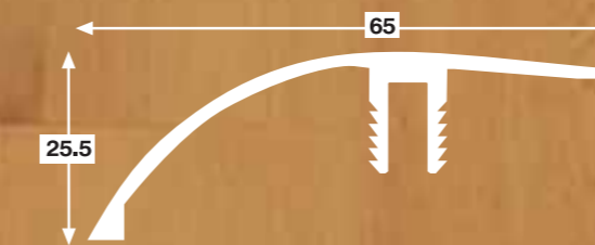
LLHR 22 RAMP
